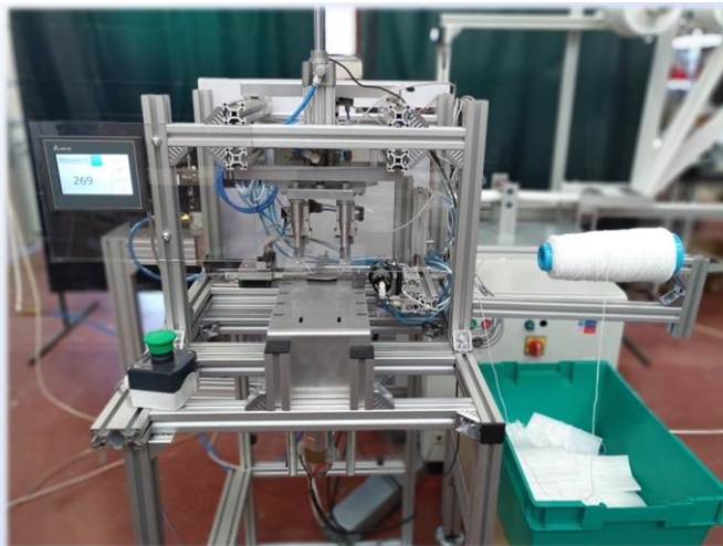
stroj na zváranie gumičiek
